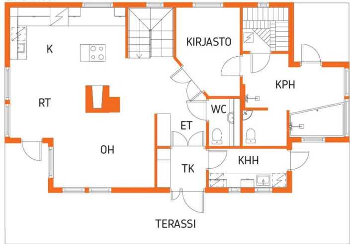
1.KERROS
